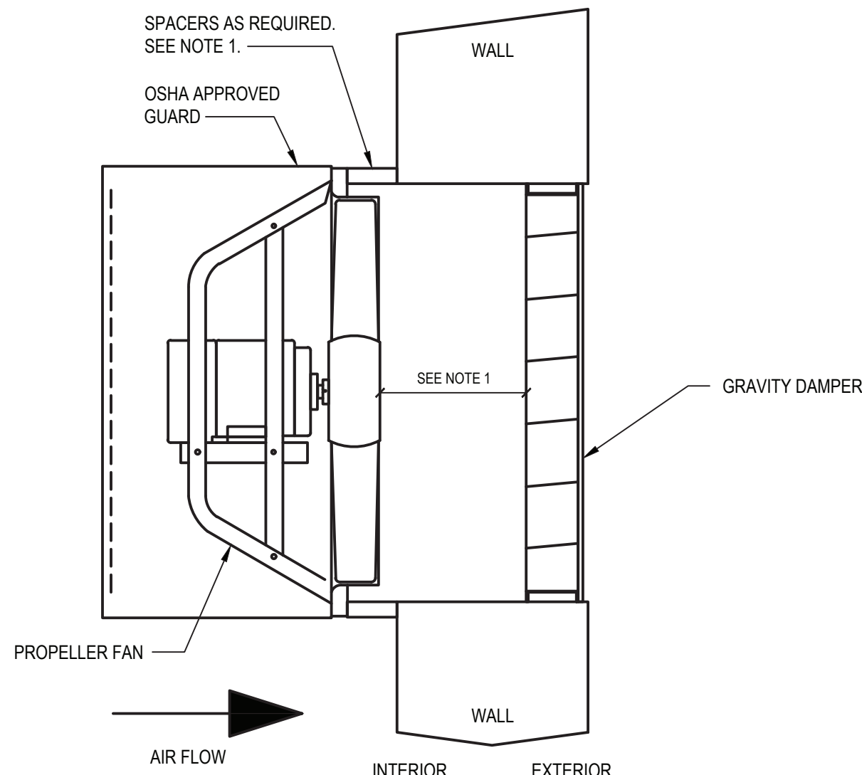
2 Sidewall Fan with OSHA Guard SCALE: NTS (DETAIL #)
