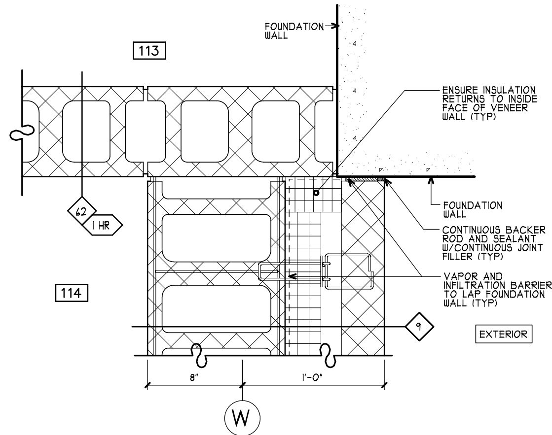
15 PLAN DETAIL (2IFLR) (2 FLR sim.) A405 SCALE: 1 1/2" = 1'-0" A100, A101
