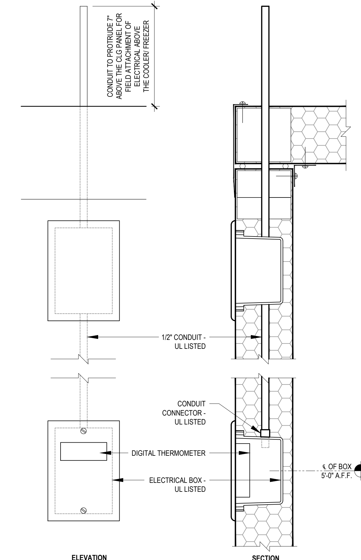
E THERMOMETER DETAIL SCALE: N.T.S.
