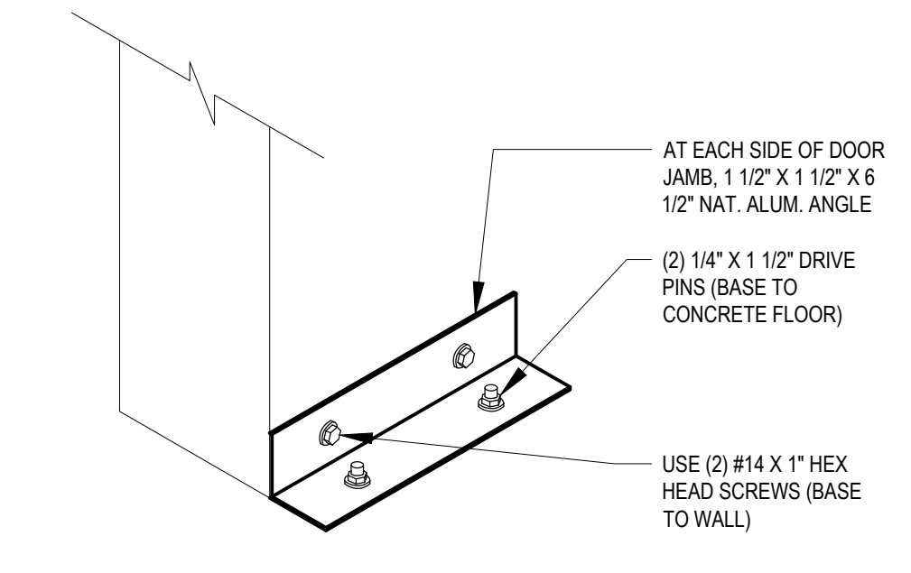
C DOOR STABILIZER DETAIL SCALE: N.T.S.
