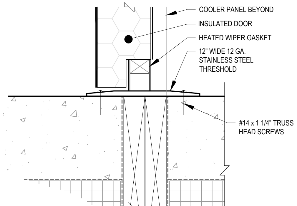
D FREEZER MAN DOOR THRESHOLD DETAIL SCALE: N.T.S.
