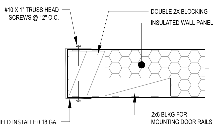
A PRODUCE AND DELI DOOR JAMB DETAIL SCALE: N.T.S.
