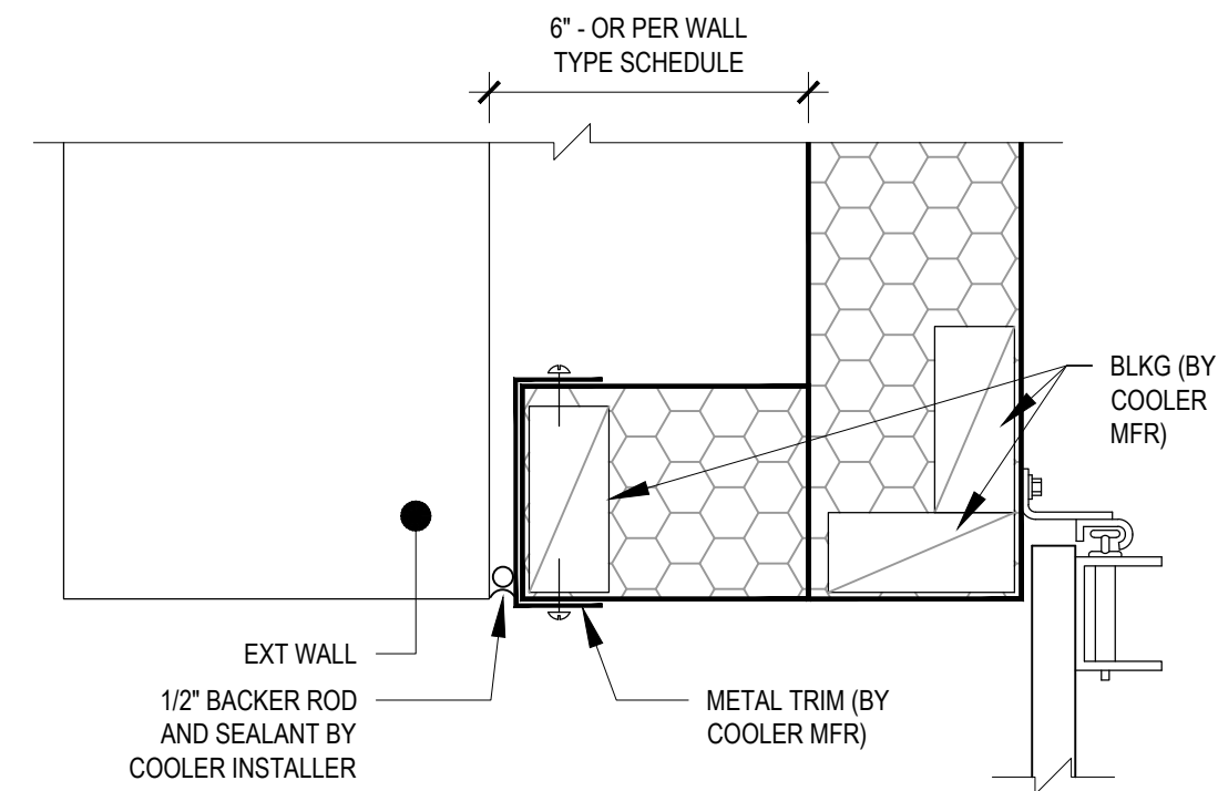
S O.H. DOOR JAMB DETAIL SCALE: N.T.S.
