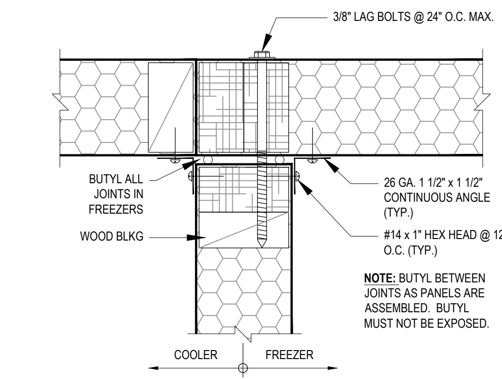
L COOLER - FREEZER CONNECTION LAG DOWN TOP DETAIL SCALE: N.T.S.
