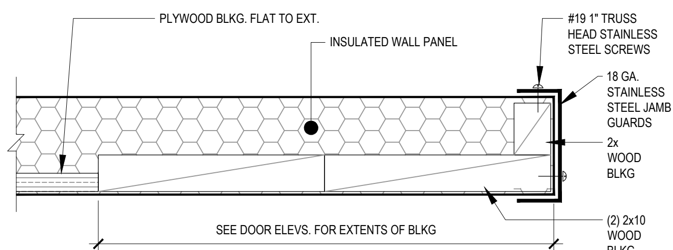
B FREEZER DOOR JAMB DETAIL SCALE: N.T.S.
