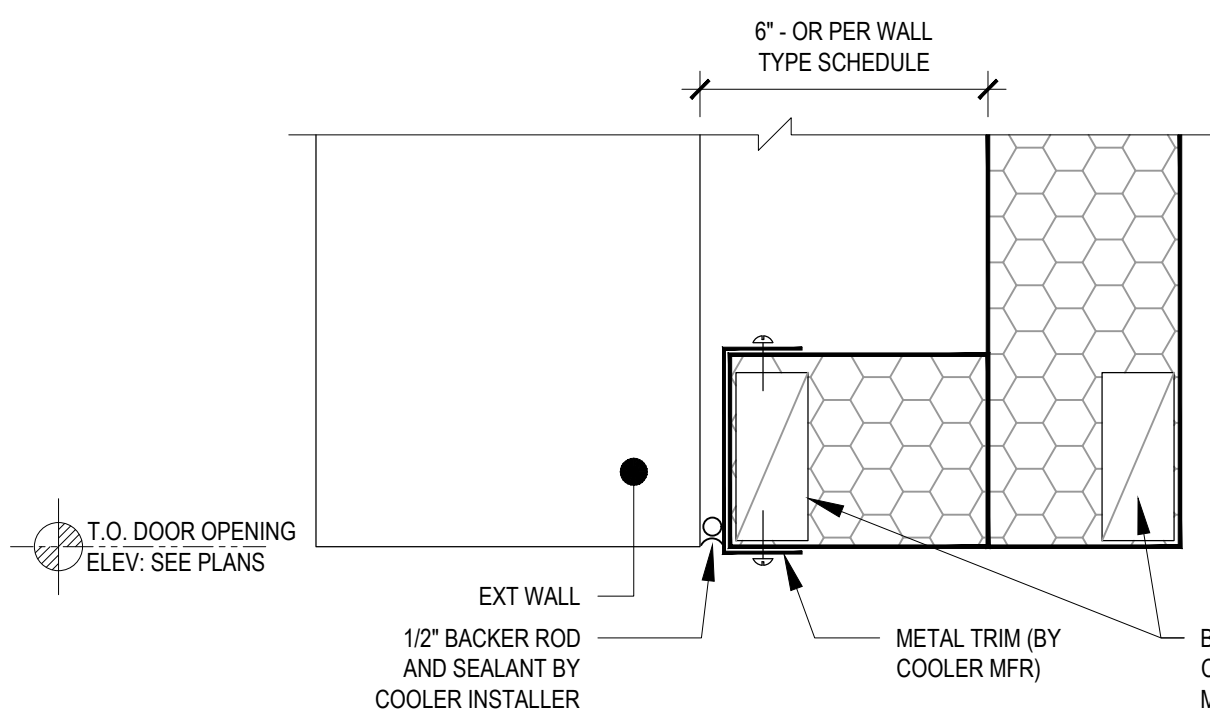
T O.H. DOOR HEAD DETAIL SCALE: N.T.S.
