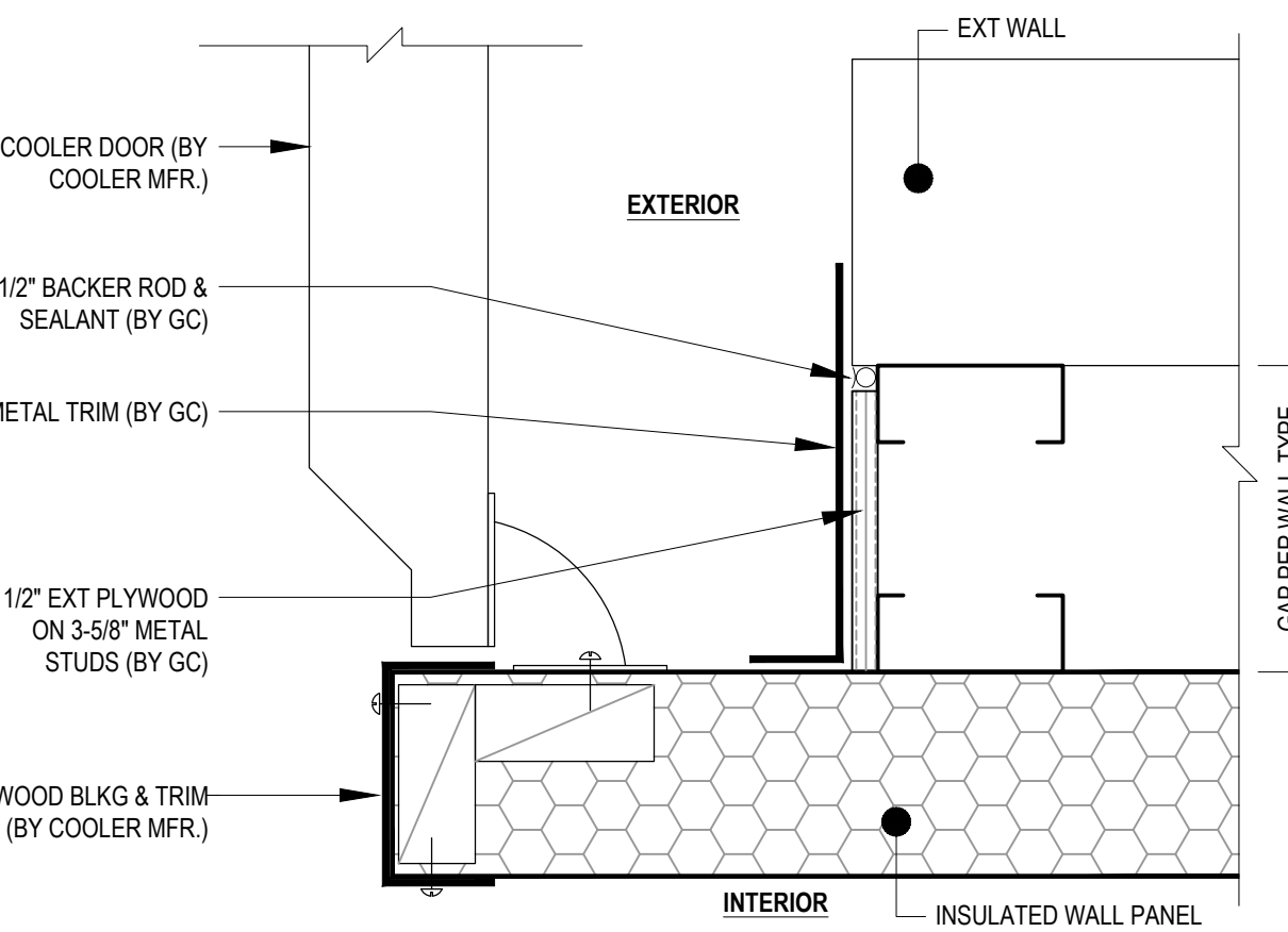
F MAN DOOR JAMB DETAIL SCALE: N.T.S.
