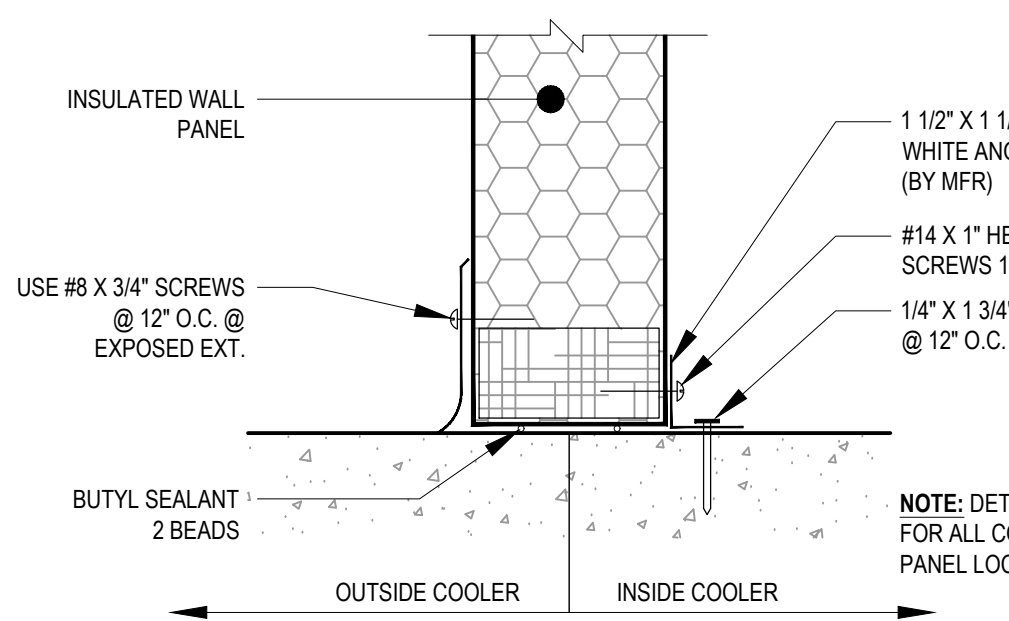
J TYP. WALL TO FLOOR DETAIL SCALE: N.T.S.
