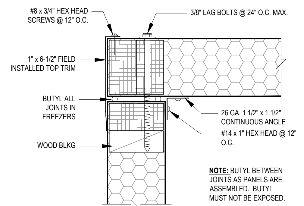
K TYP. LAG DOWN TOP DETAIL SCALE: N.T.S.
