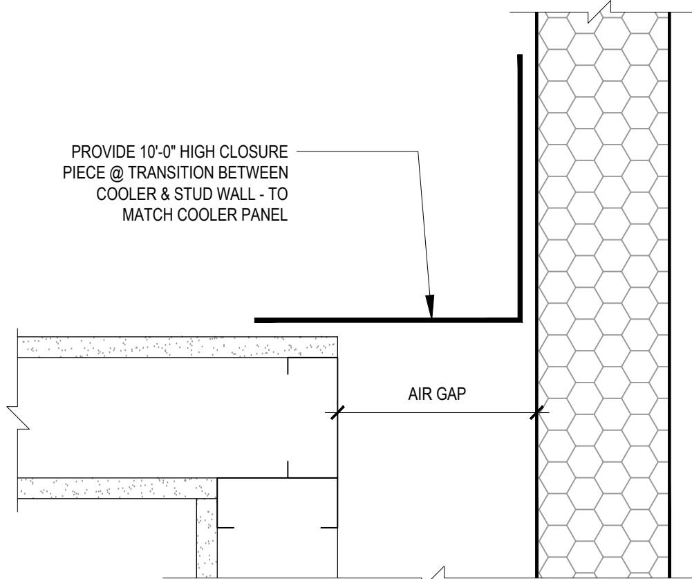
P WALL TRANSITION TRIM DETAIL SCALE: N.T.S.
