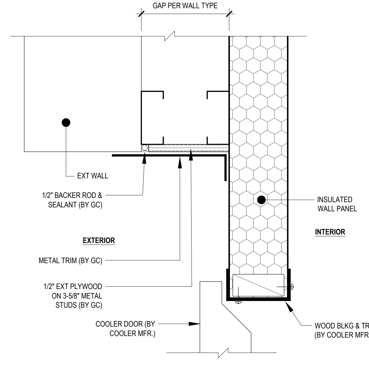
G MAN DOOR HEAD DETAIL SCALE: N.T.S.
