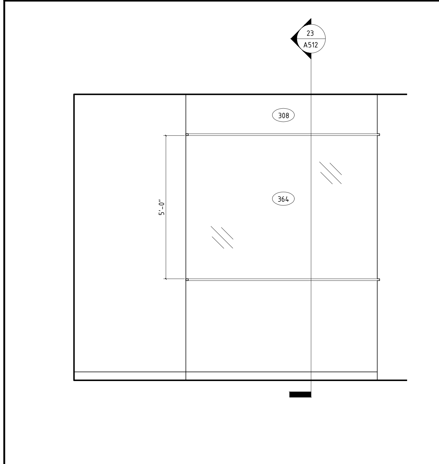
33 SHELVING DISPLAY ELEVATION A512 SCALE: 1/2" = 1'-0"
