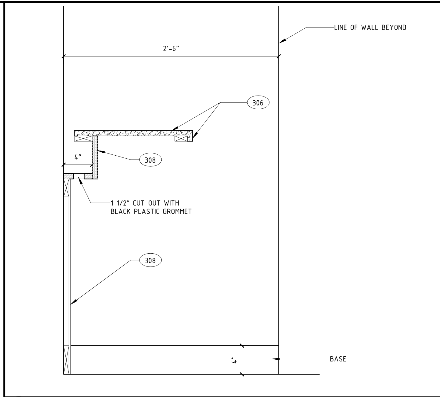
31 QUICK PRINT SECTION A512 SCALE: 1 1/2" = 1'-0"
