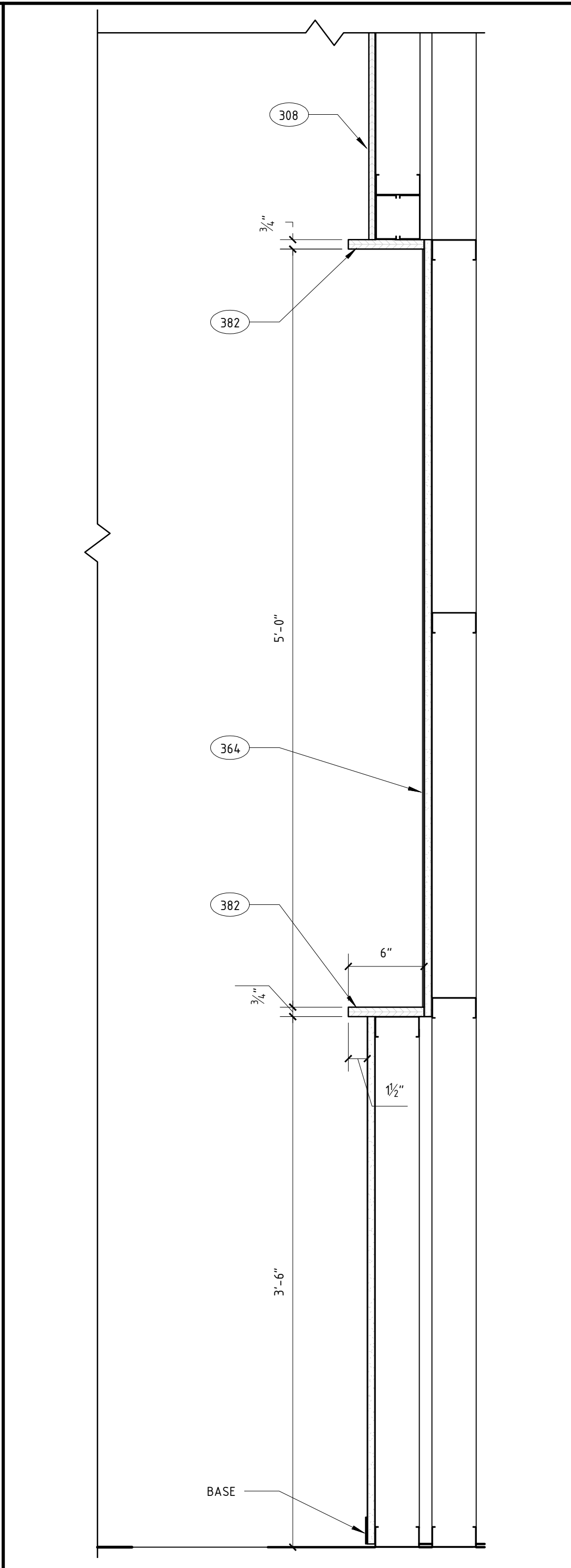
23 SHELVING DISPLAY SECTION A512 SCALE: 1/2" = 1'-0"
