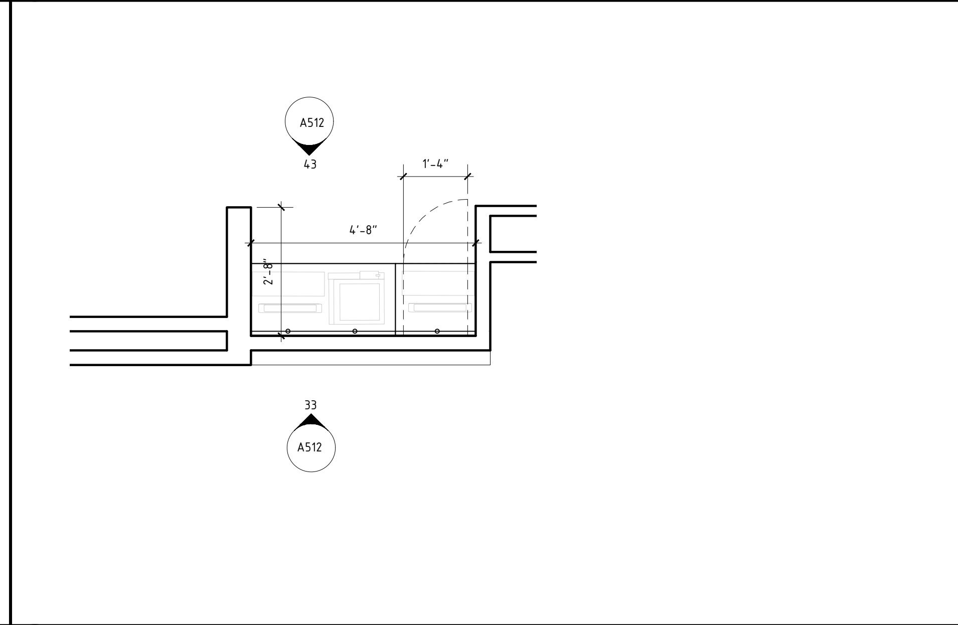
44 QUICK PRINT PLAN A512 SCALE: 1/2" = 1'-0"
