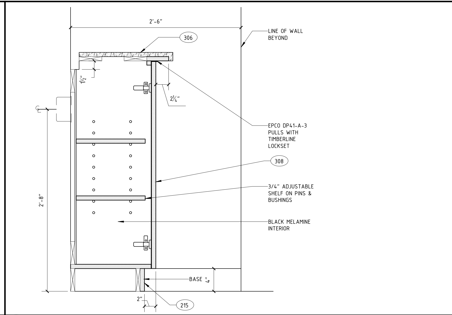
41 QUICK PRINT SECTION A512 SCALE: 1 1/2" = 1'-0"
