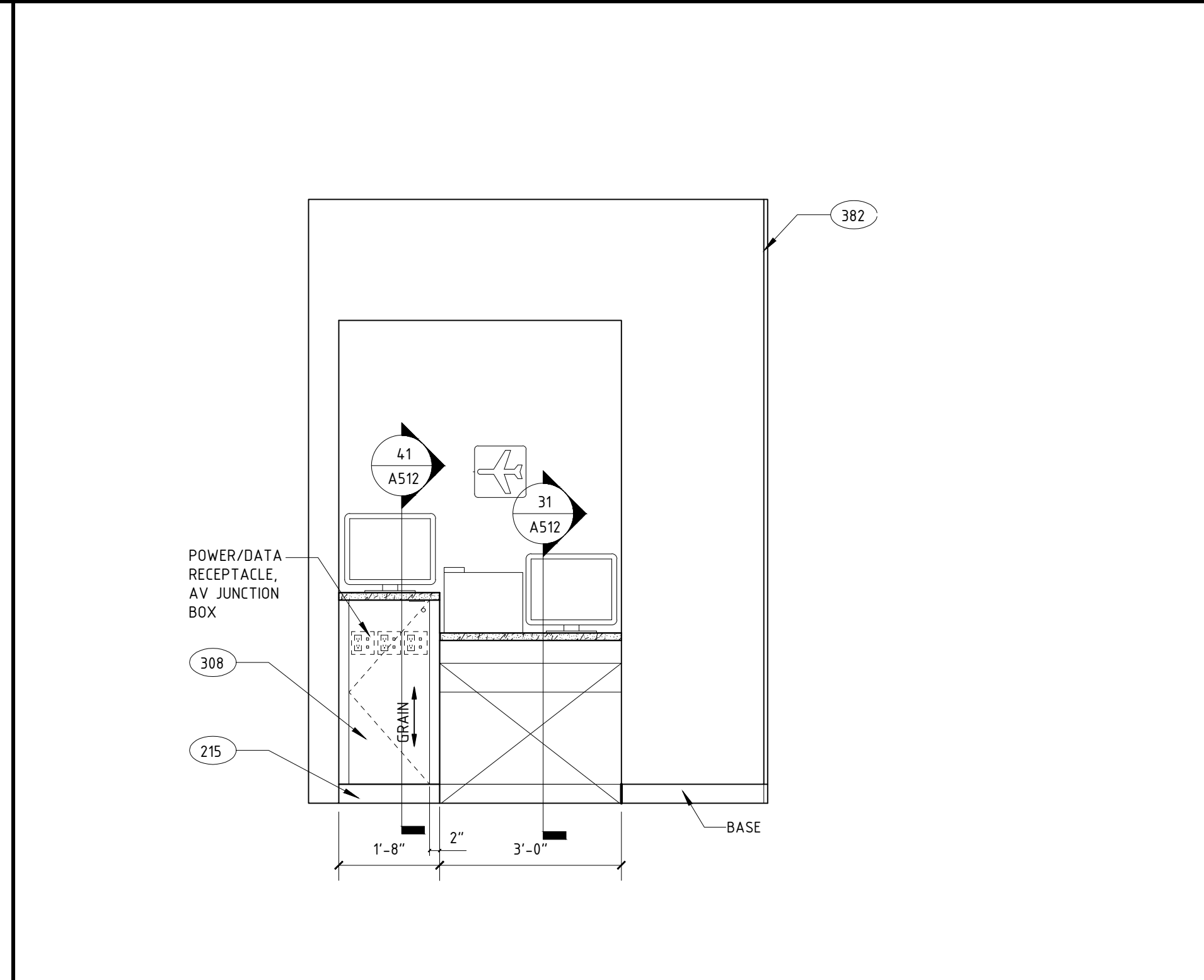
43 QUICK PRINT ELEVATION A512 SCALE: 1/2" = 1'-0"
