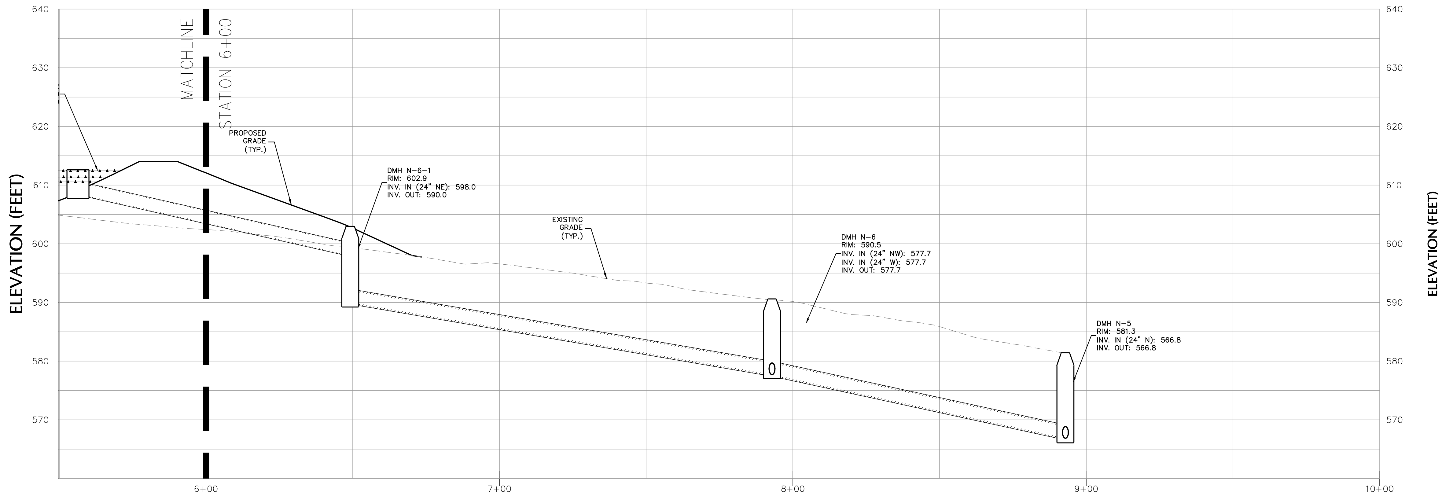
BASIN 4A-1-B HORIZONTAL SCALE: 1" = 20' VERTICAL SCALE: 1" = 10'
