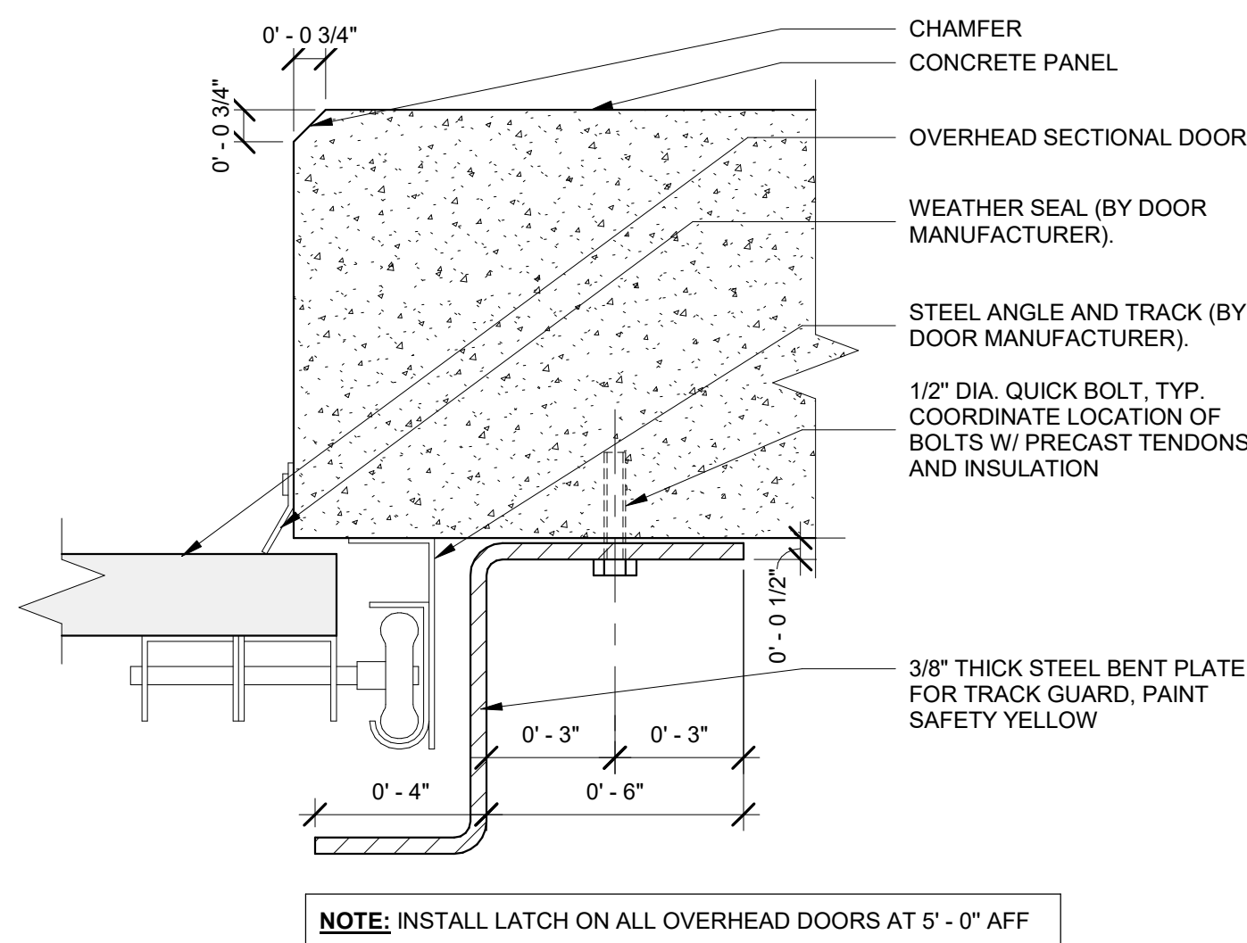
SECTIONAL DOOR JAMB
