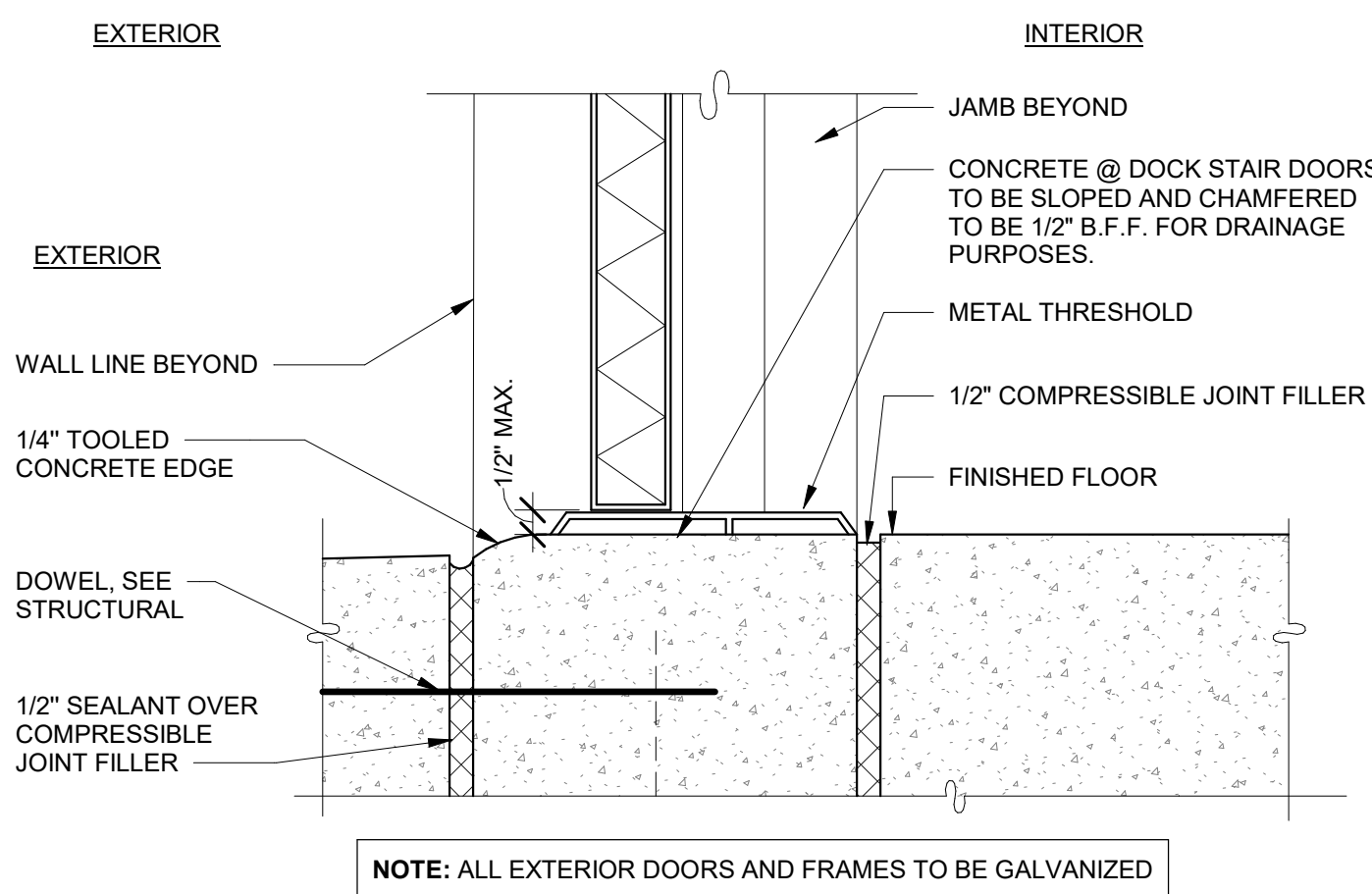
HOLLOW METAL DOOR SILL
