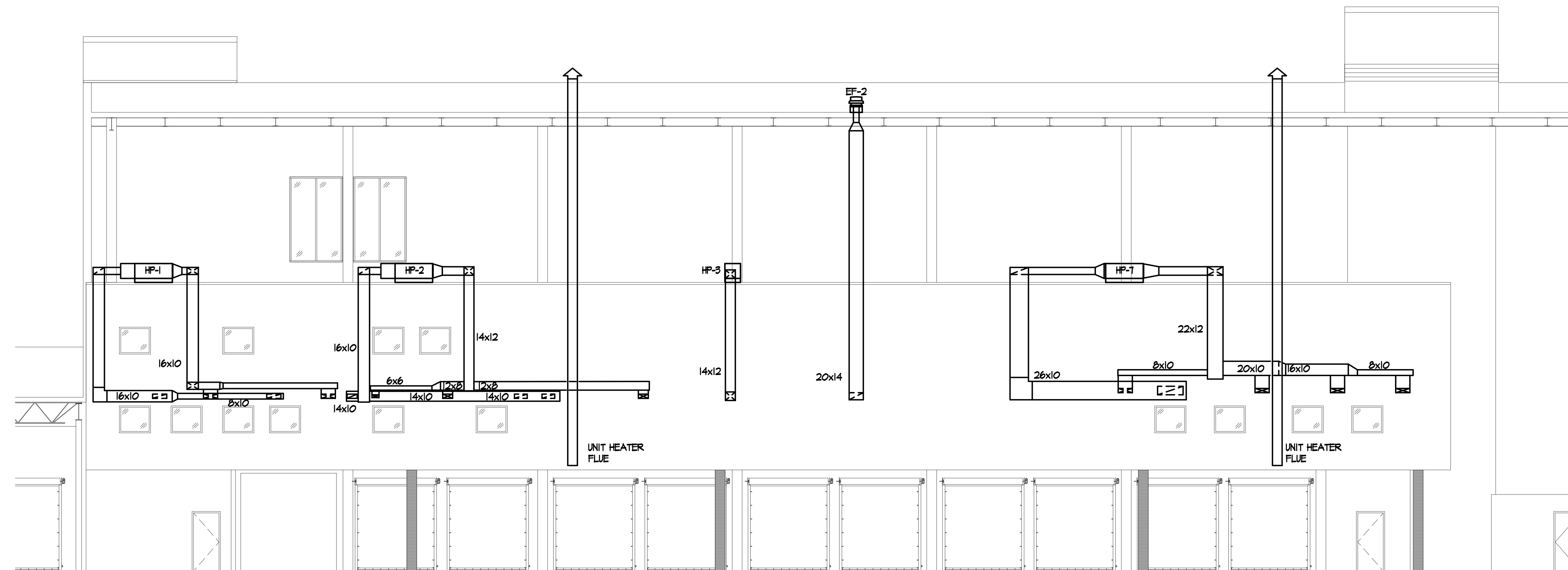
MEZZANINE ELEVATION SCALE: 1/8"=1'-0"
