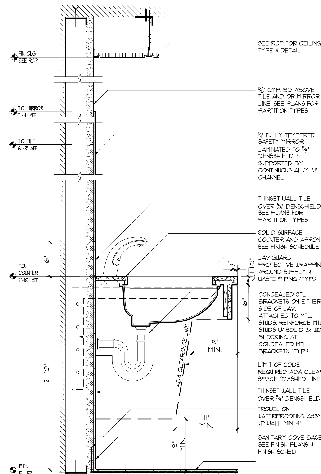
16 SECTION DETAIL SCALE: 1-1/2"=1'-0"
