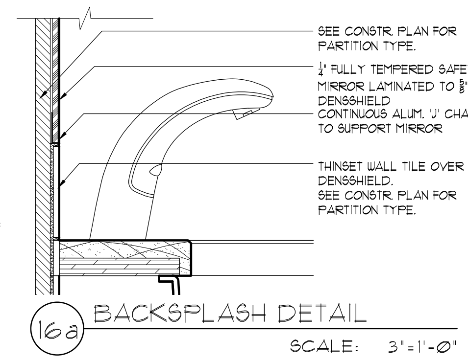
16a BACKSPASH DETAIL SCALE: 3"=1'-0"
