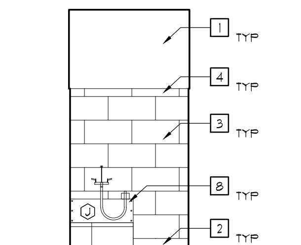
15 JANITOR CL. ELEV. SCALE: 1/4"=1'-0"
