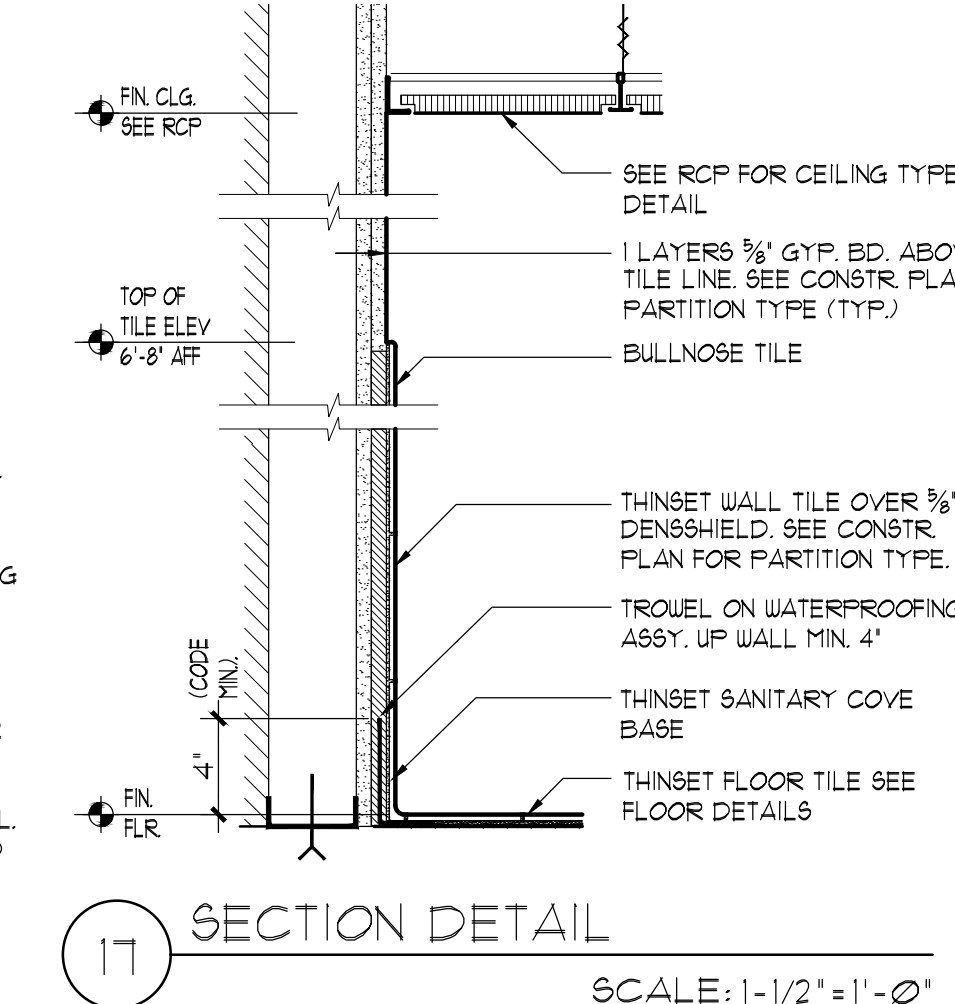
17 SECTION DETAIL SCALE: 1-1/2"=1'-0"
