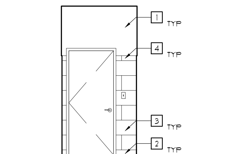
13 JANITOR CL. ELEV. SCALE: 1/4"=1'-0"
