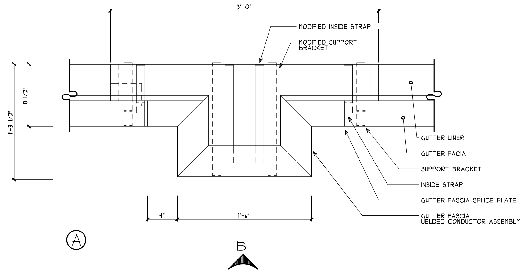
2 COLLECTION BOX DETAIL A-106 SCALE: 1-1/2" = 1'-0"
