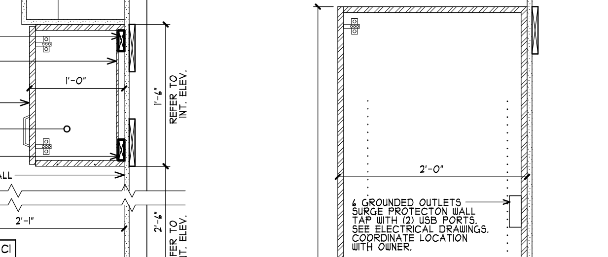
14 RADIO ROOM CONSOLE A130 SCALE: 1" = 1'-0" 5/A110
