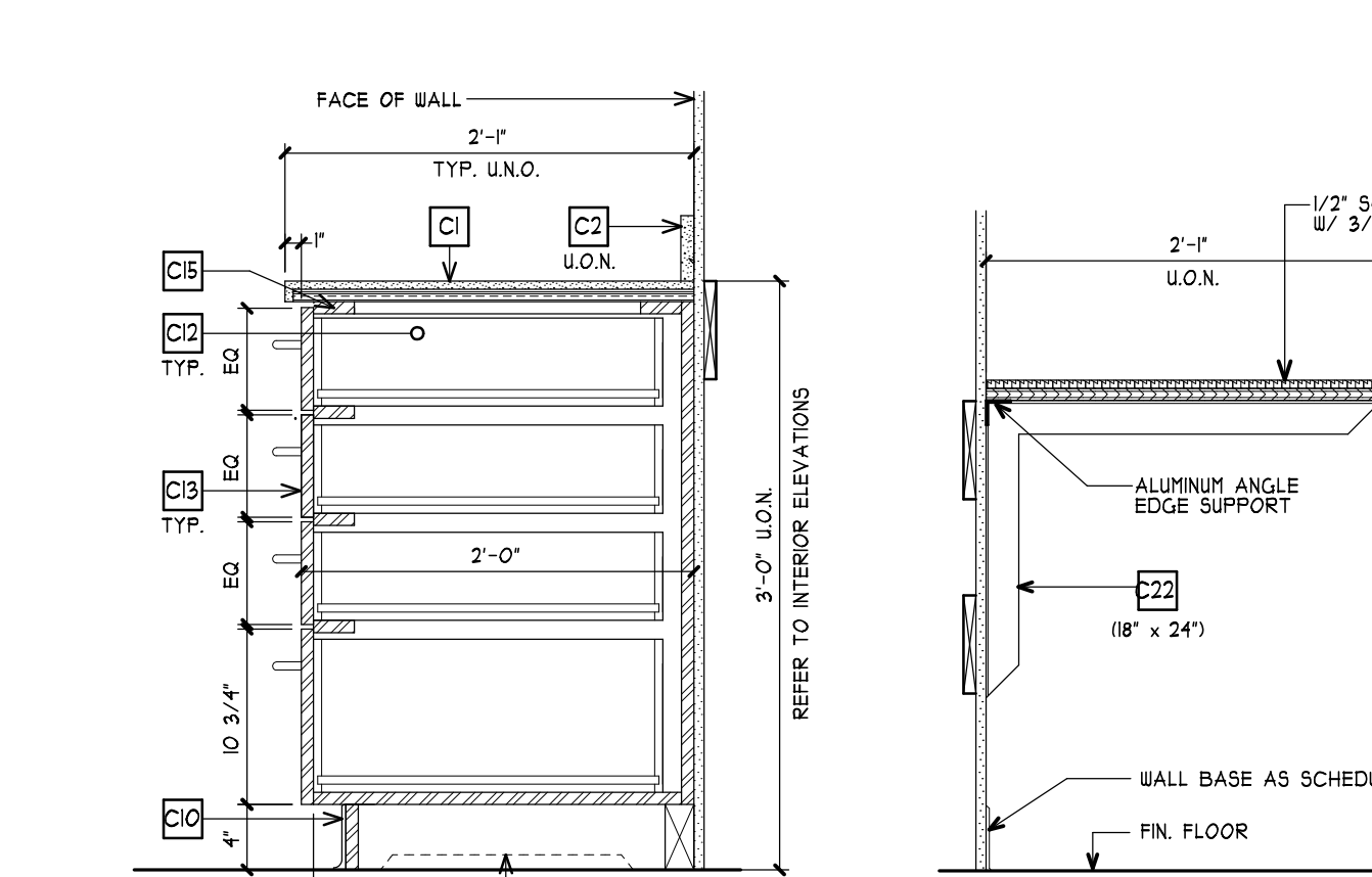
9 DISPLAY CASE A130 SCALE: 1" = 1'-0" 1/A100 & 1/A102
