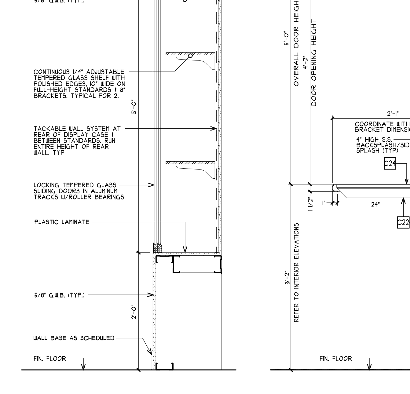
9 DISPLAY CASE A130 SCALE: 1" = 1'-0" 1/A100 & 1/A102
