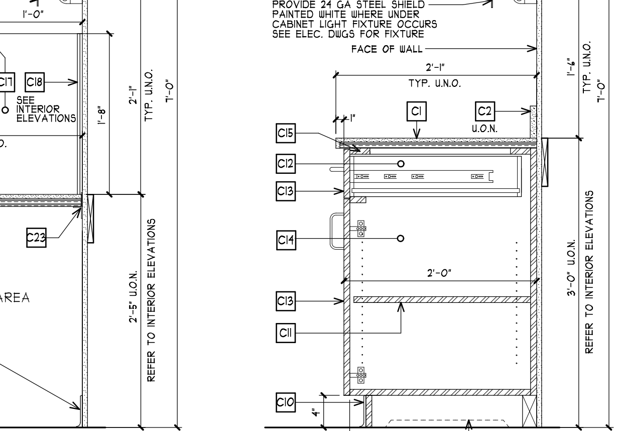
9 DISPLAY CASE A130 SCALE: 1" = 1'-0" 1/A100 & 1/A102
