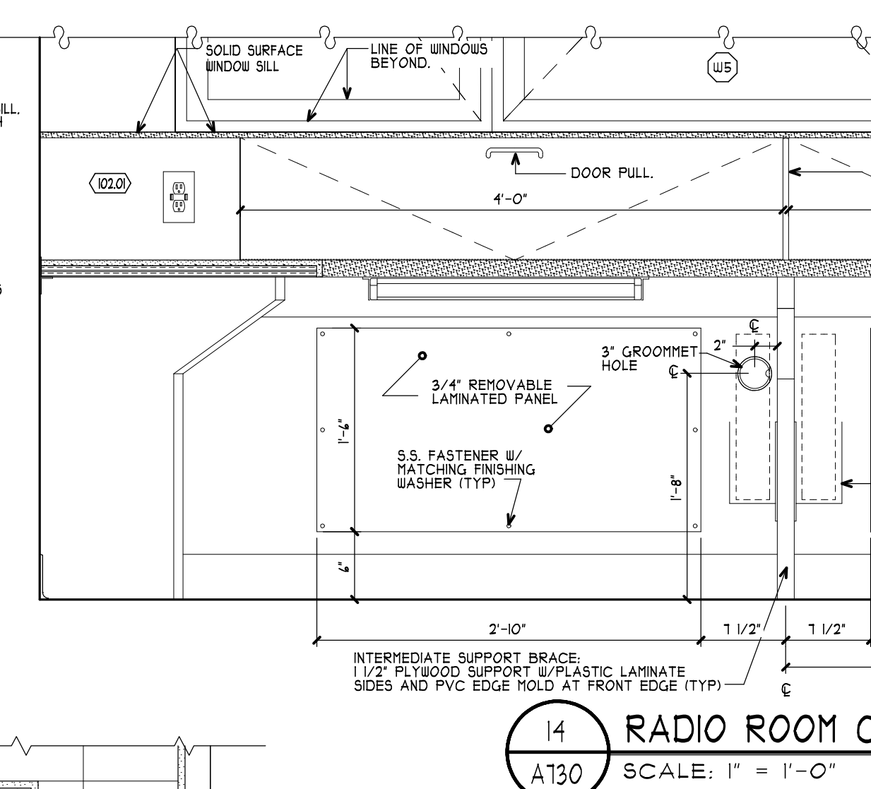
14 RADIO ROOM CONSOLE A130 SCALE: 1" = 1'-0" 5/A110
