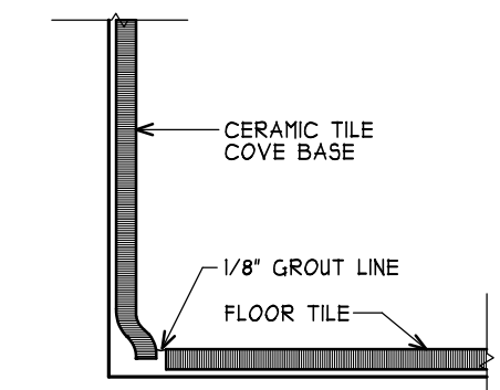
5 CERAMIC TILE COVE BASE SCALE: 3" = 1'-0"
