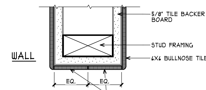
2 CERAMIC TILE END WALL SCALE: 3" = 1'-0"
