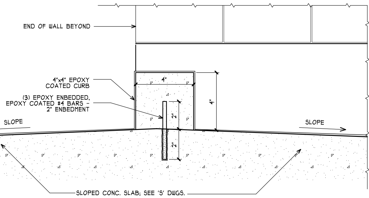
2 SHOWER FLOOR TRANSITION SCALE: N.T.S. 1/A800
