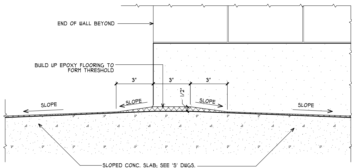
3 SHOWER FLOOR TRANSITION SCALE: N.T.S. 1/A800
