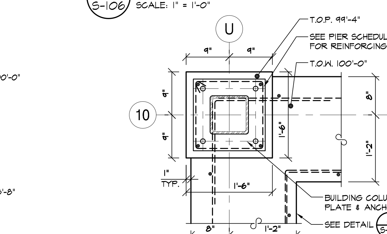
9 DETAIL S-106 SCALE: 1" = 1'-0"
