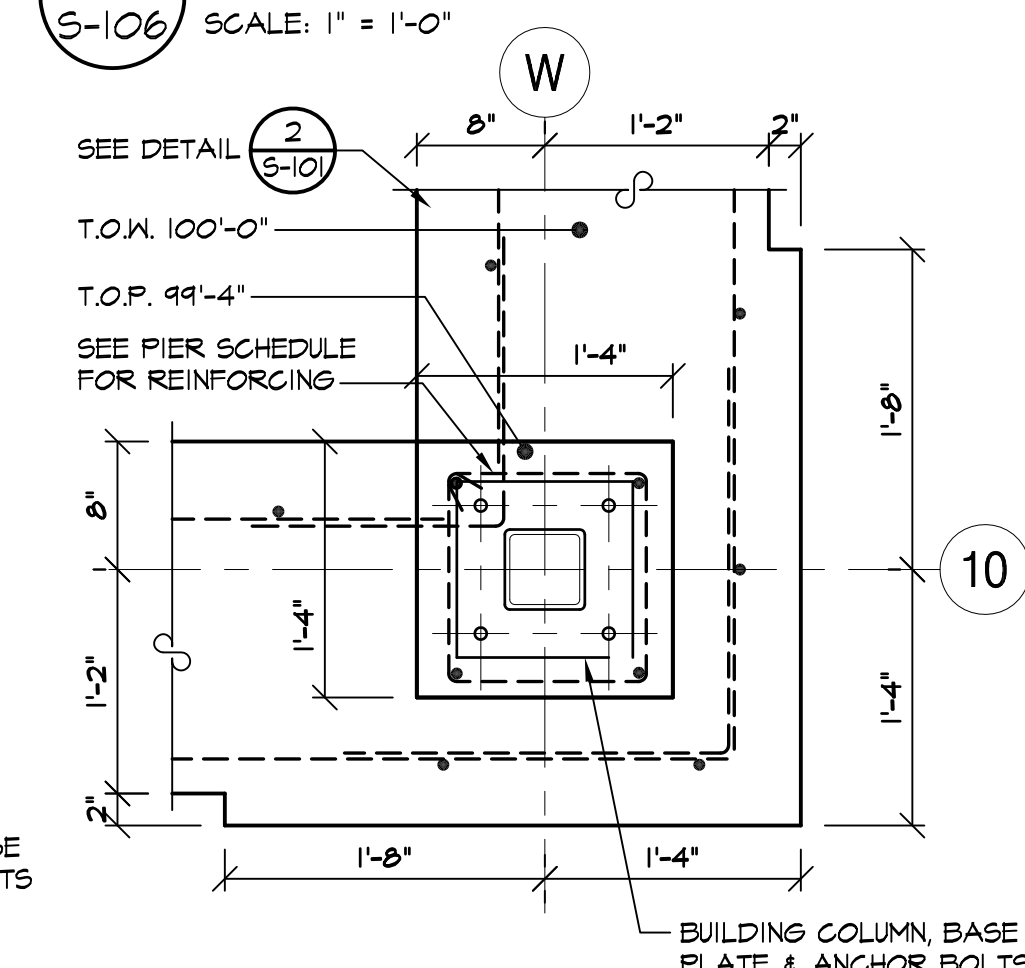
10 DETAIL S-106 SCALE: 1" = 1'-0"
