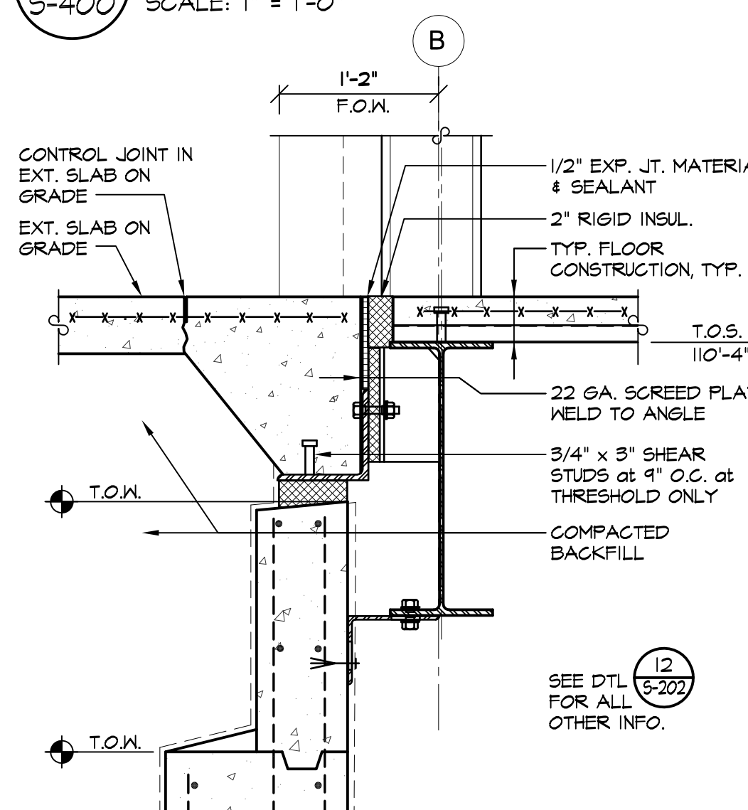
2 HIGH SEC. FL THRESHOLD S-400 SCALE: 1" = 1'-0"
