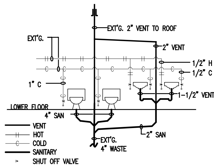
8 PLUMBING RISER DIAGRAM N.T.S.
