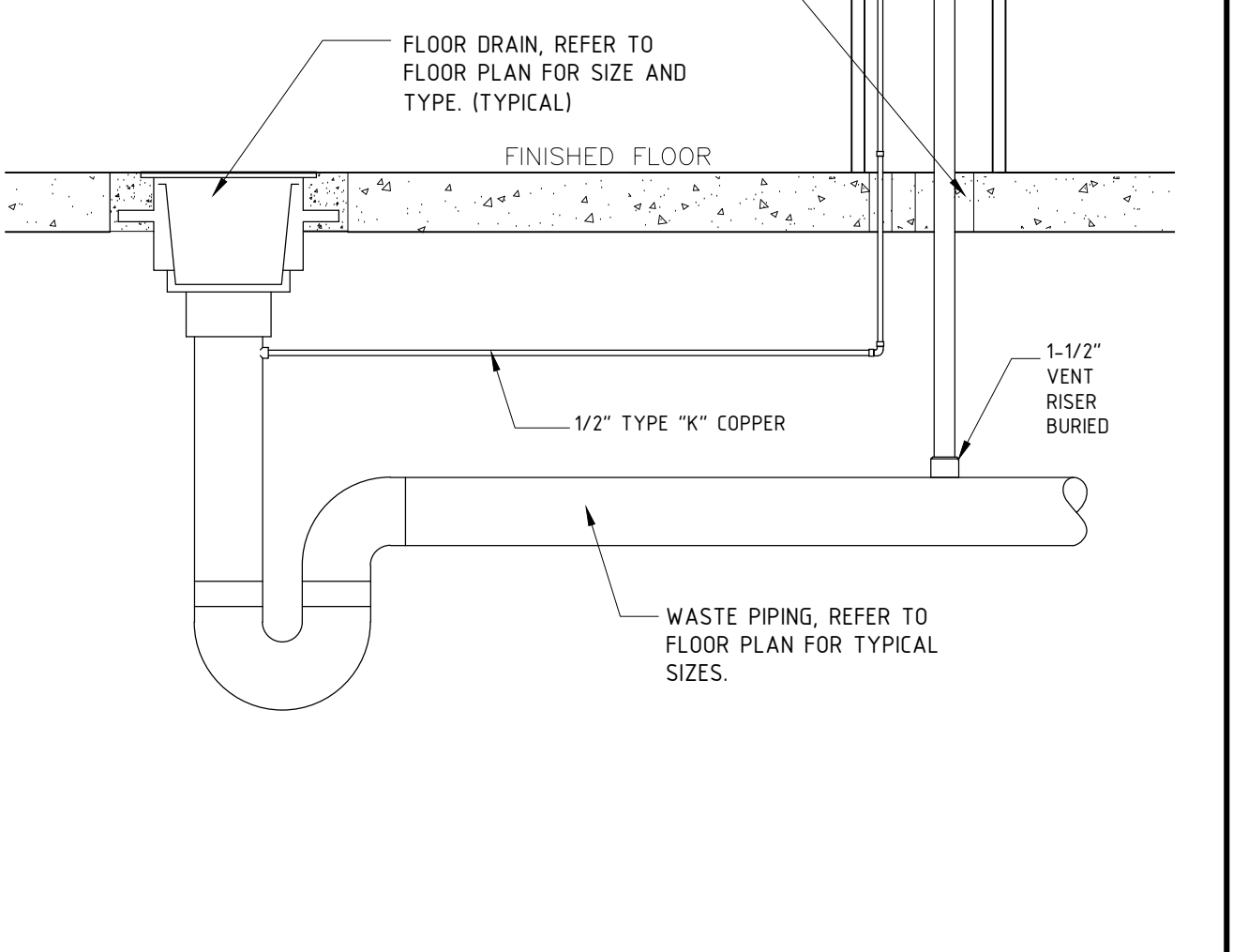
34 TRAP PRIMER SECTION
