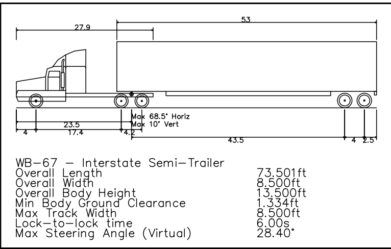
WB-67 PROFILE SCALE: N.T.S.
