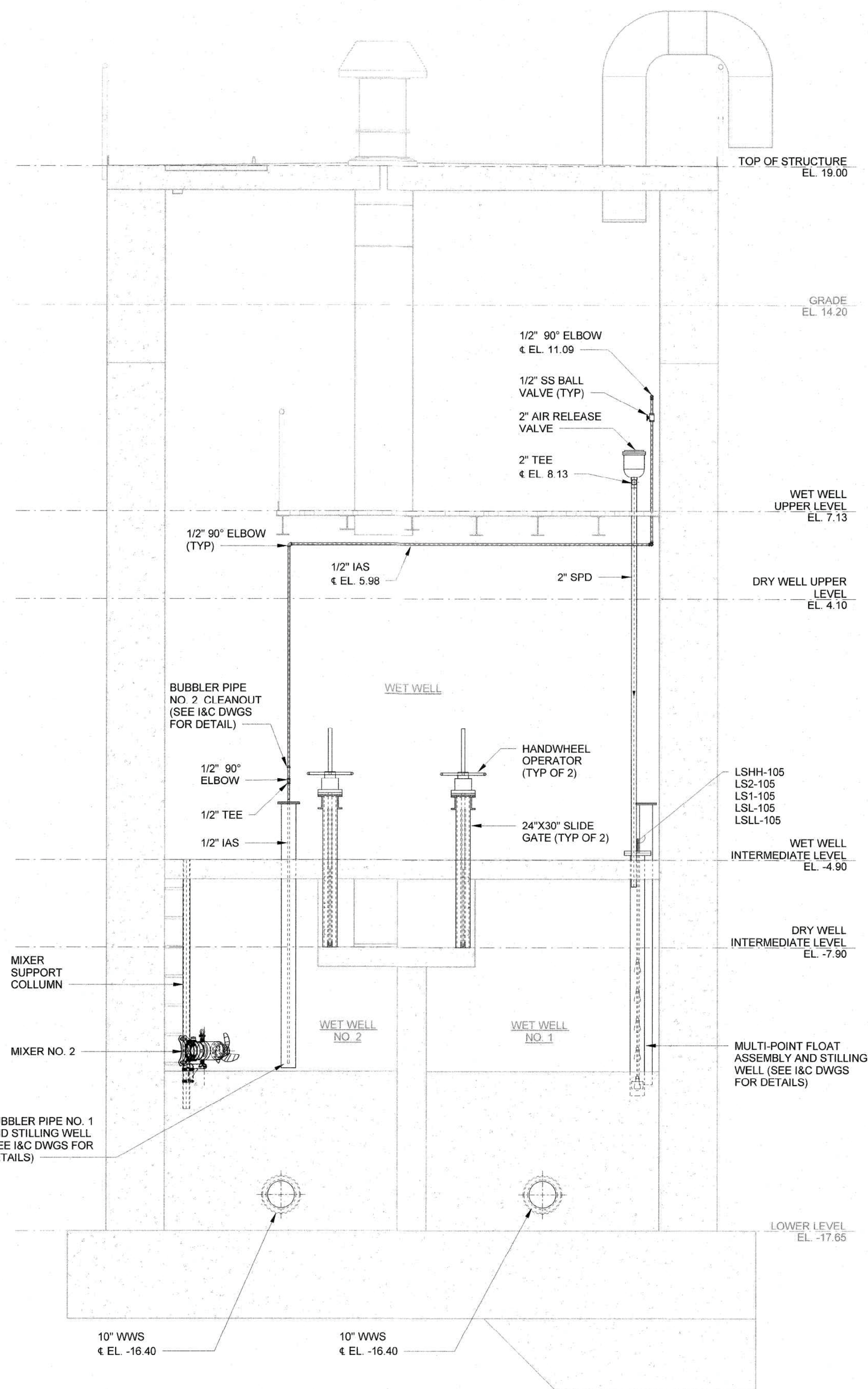
1 SECTION M-009 SCALE: 3/8" = 1'-0"
