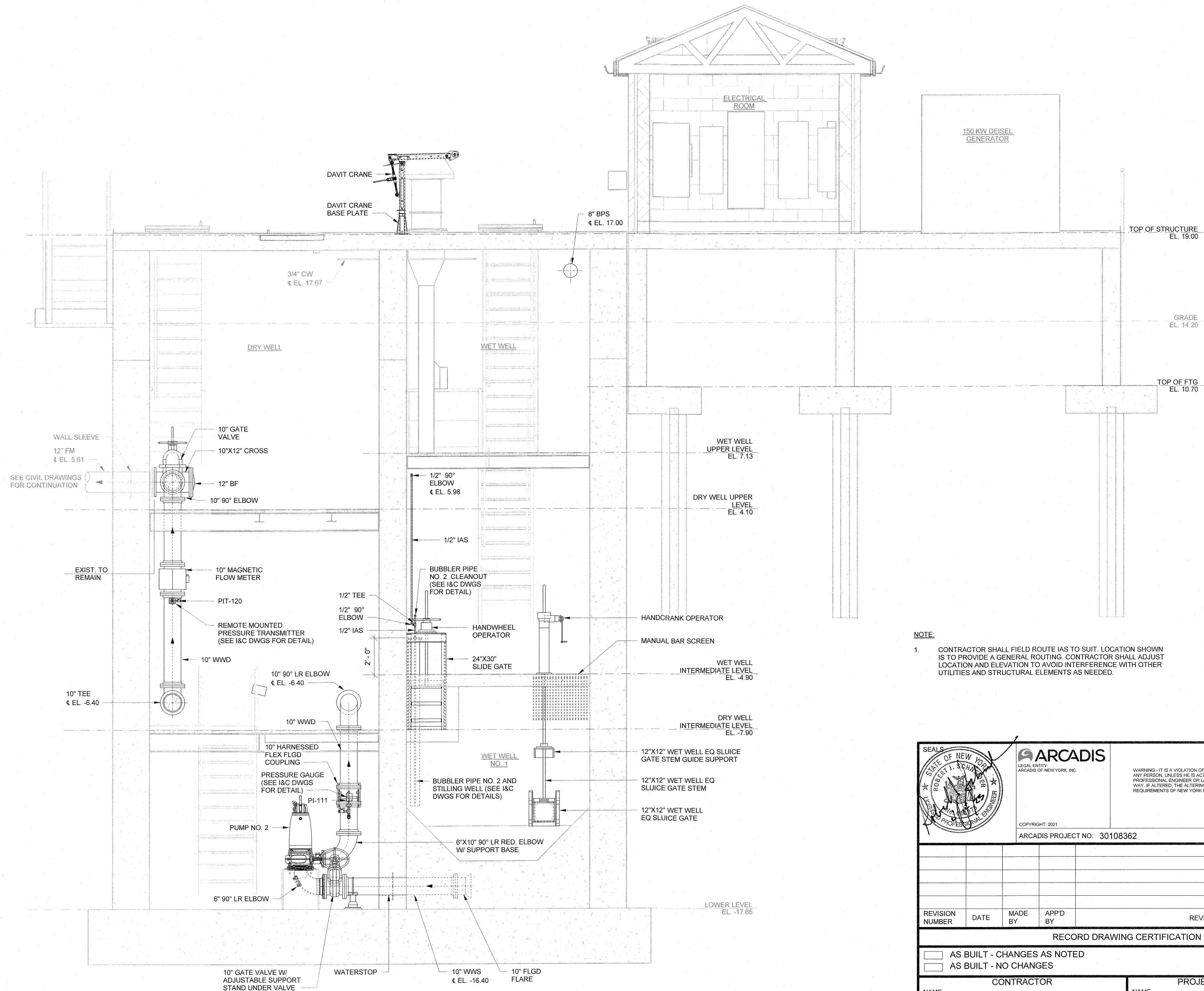
1 SECTION M-009 SCALE: 3/8" = 1'-0"
