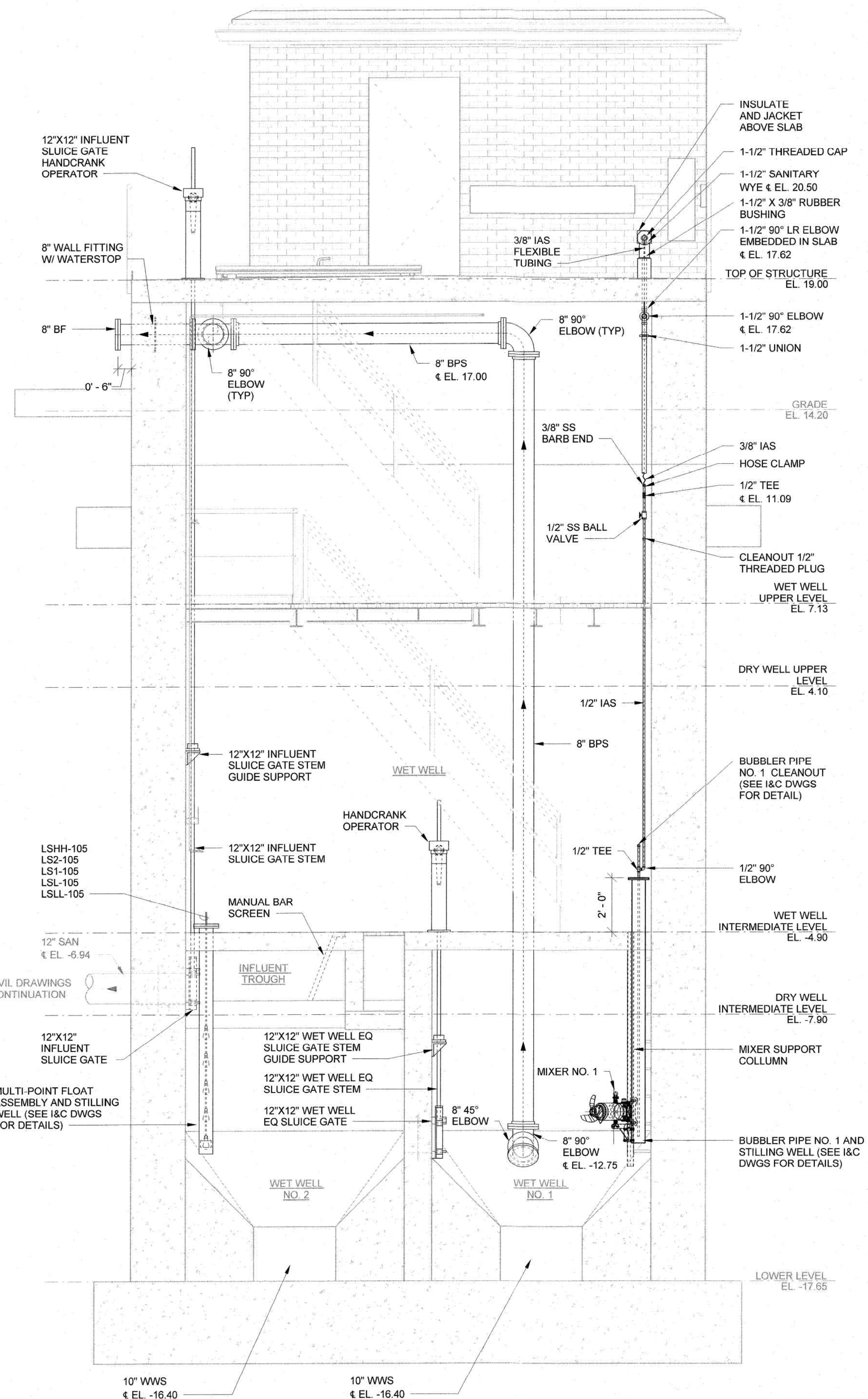
2 SECTION M-009 SCALE: 3/8" = 1'-0"
