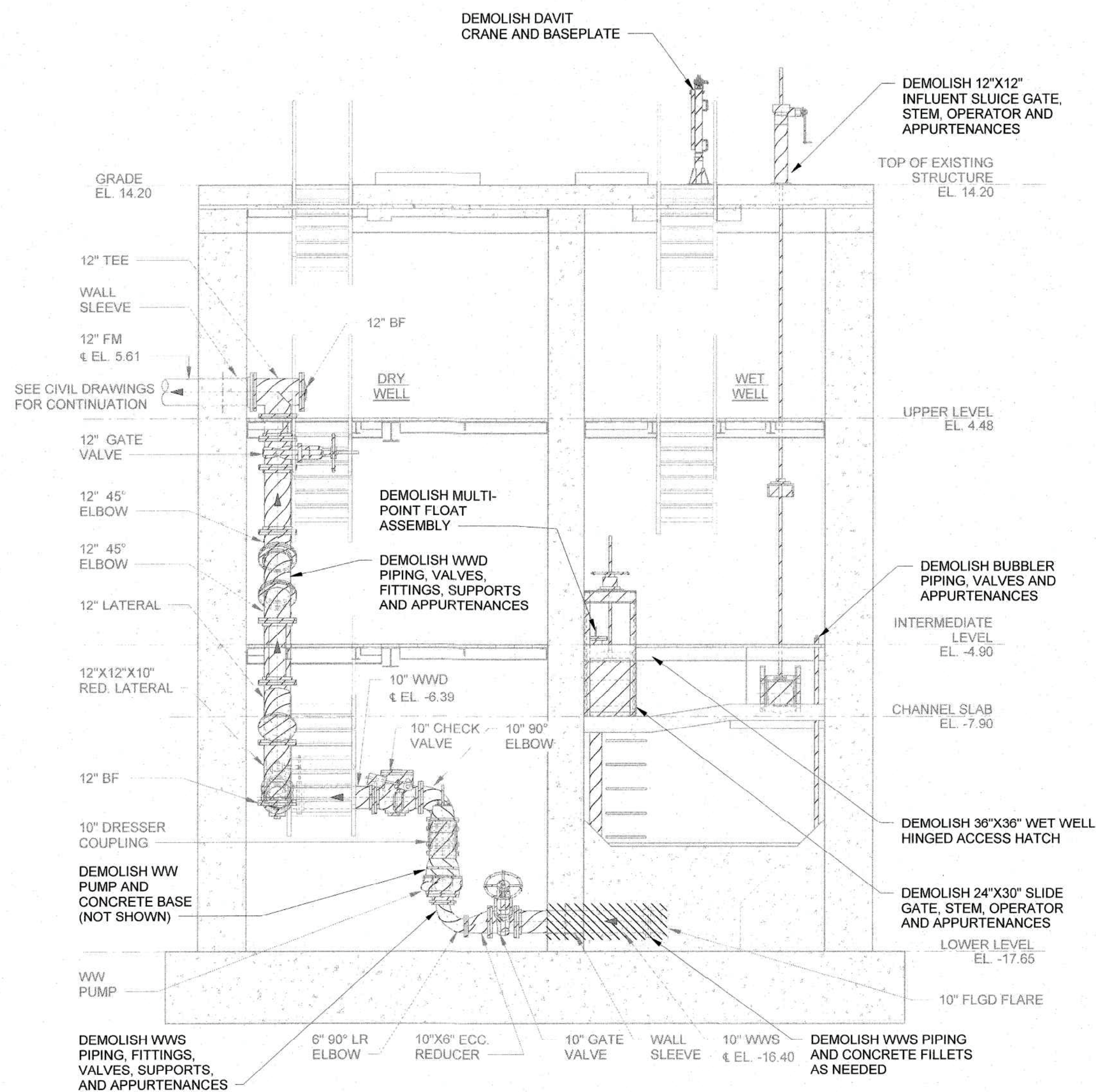
2 SECTION M-002 SCALE: 1/4" = 1'-0"
