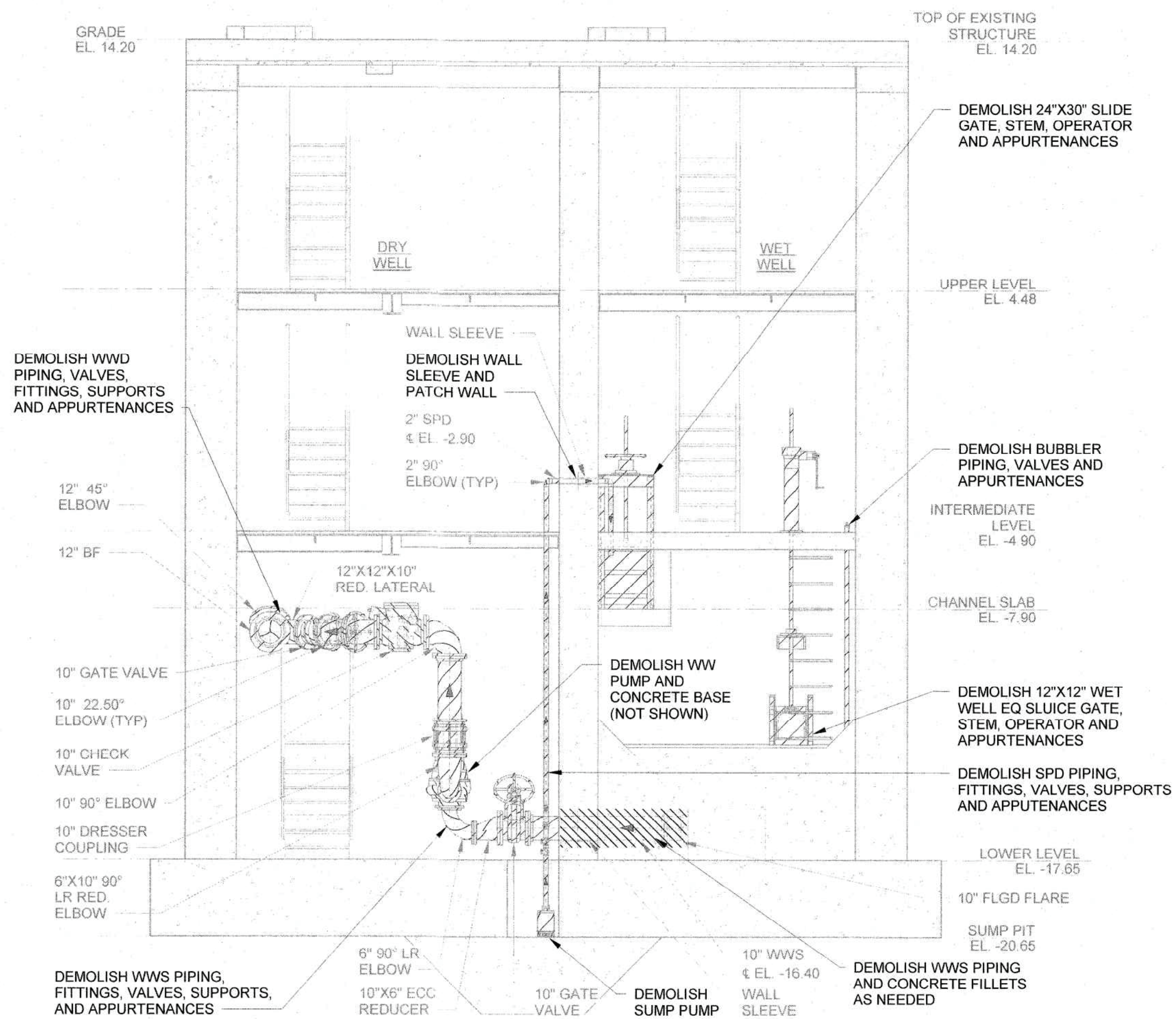
1 SECTION M-002 SCALE: 1/4" = 1'-0"
