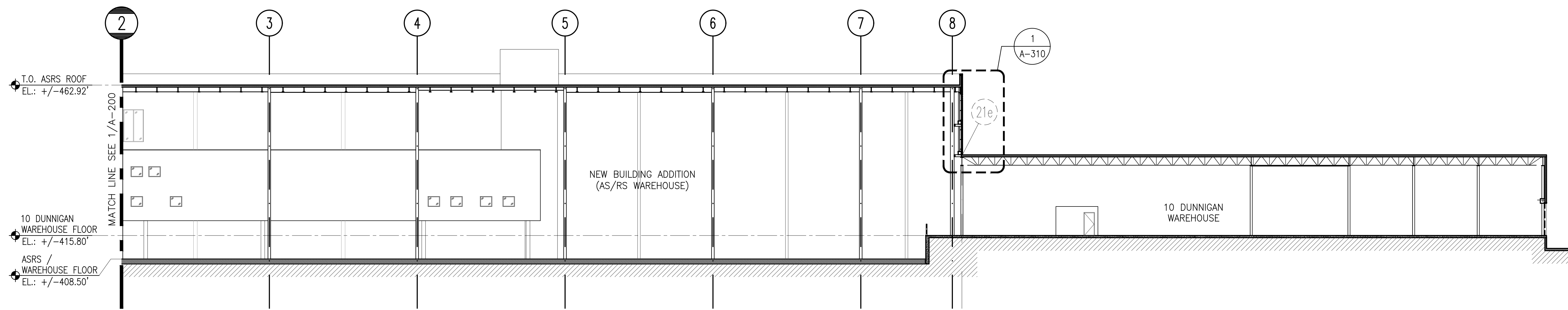
2 BUILDING SECTION - LONGITUDINAL 1B A-101 A-200 SCALE: 1/16"=1'-0" 0 8 16 32 FT
