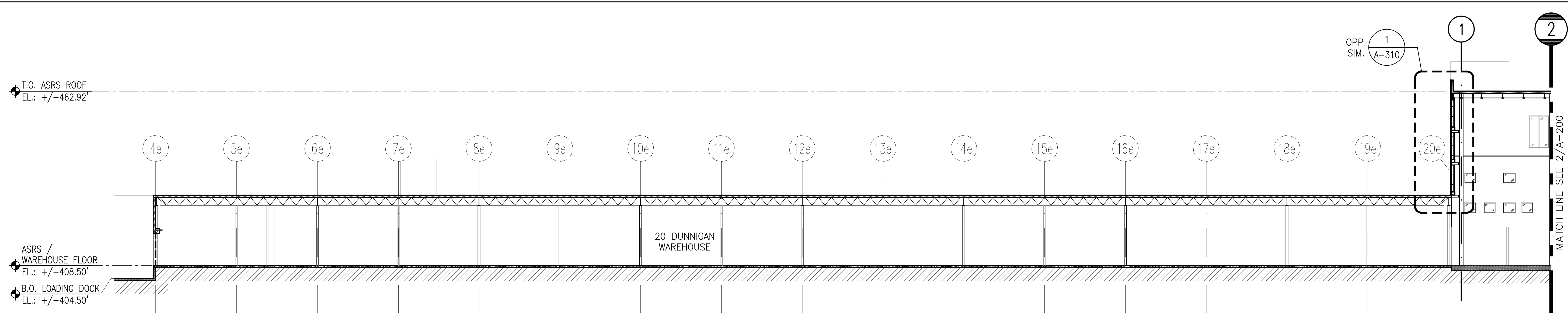
1 BUILDING SECTION - LONGITUDINAL 1A A-101 A-200 SCALE: 1/16"=1'-0" 0 8 16 32 FT
