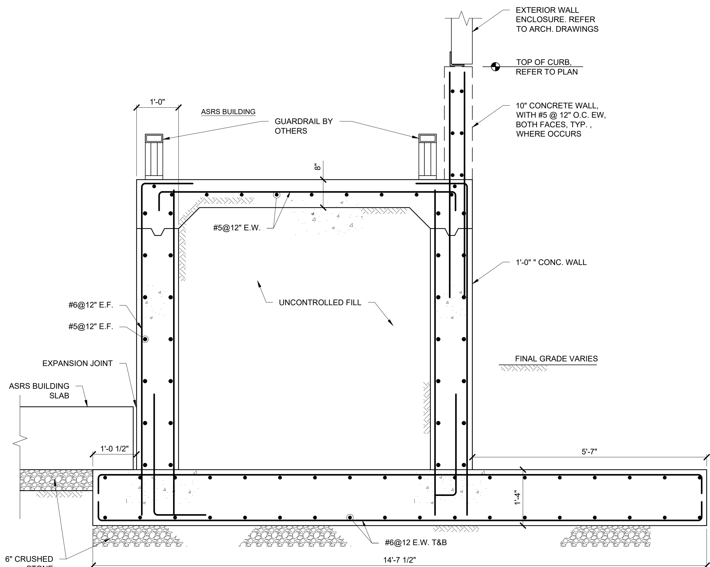
K SECTION SCALE: 3/4" = 1'-0"
