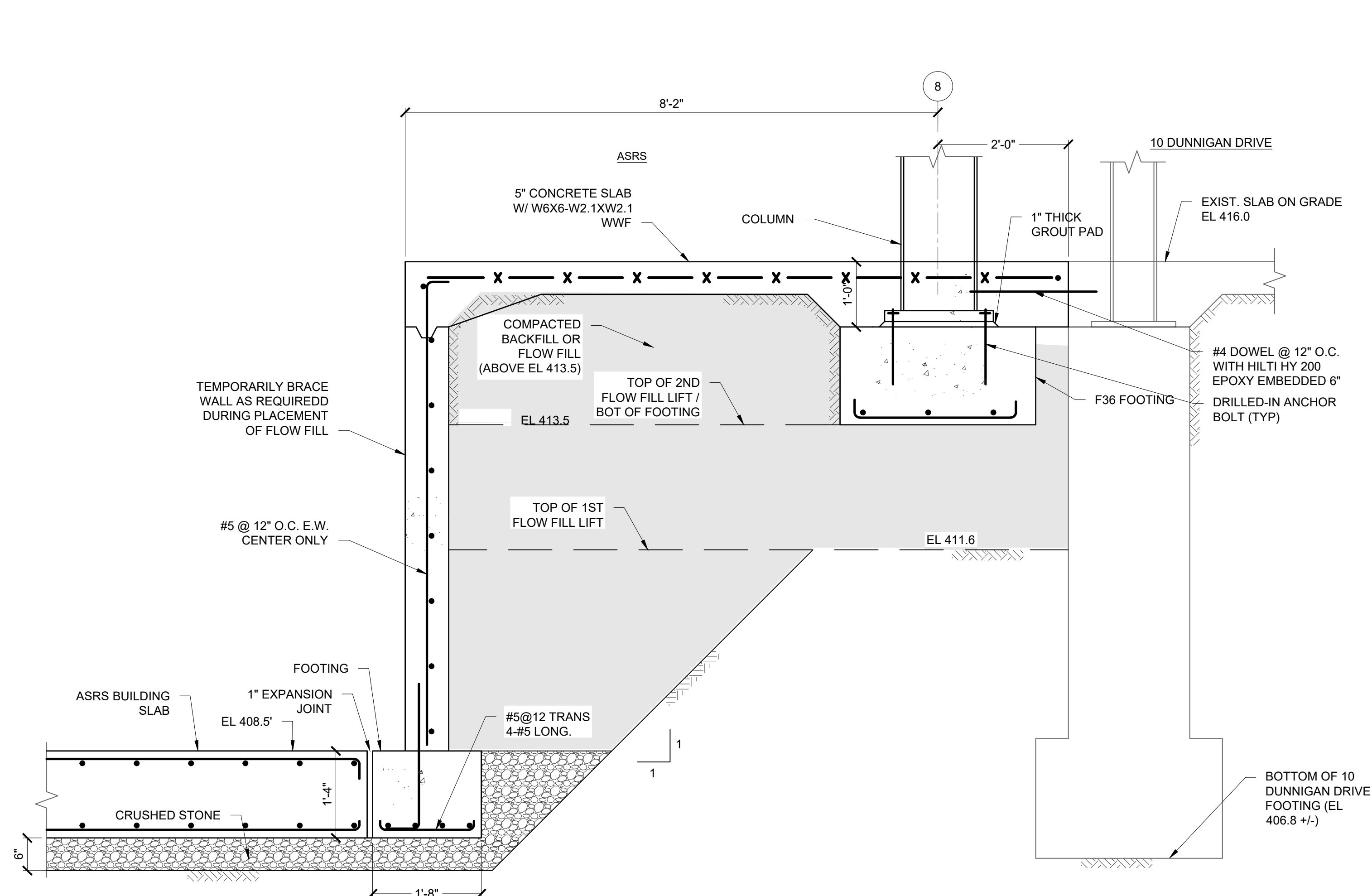
L SECTION SCALE: 3/4" = 1'-0"
