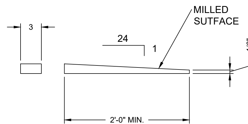
TYPICAL WEDGE DETAIL SCALE: N.T.S.
