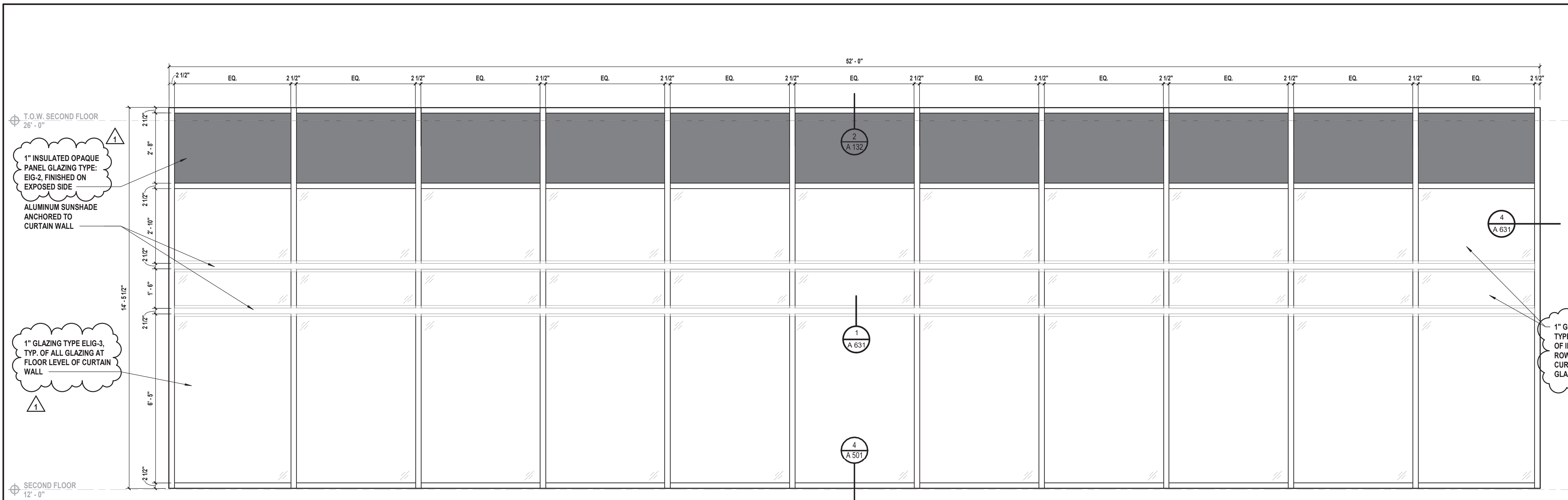
L Curtain Wall Type L SCALE: 1/2" = 1'-0"
